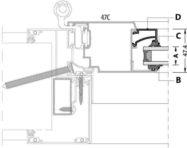
GLAZING TABLE / CAM TABLOSU
